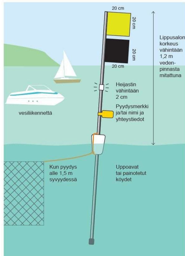
Kuva 2. Pintapyydys eli lähemmäksi kuin 1,5 metriä veden pintaa ulottuva pyydys, tulee vesiliikenteen käyttämillä alueilla merkitä kahdella päällekkäin kiinnitetyllä lipulla. (Piiros Anu Väitalo/KKL)
