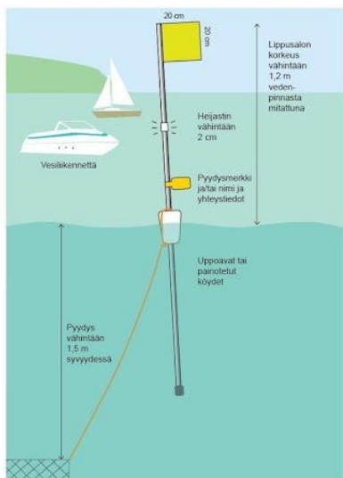
Kuva 1. Vesiliikenteen käyttämällä alueilla pyydys on merkittävä 1,2 metriä vedenpinnan yläpuolelle ulottuvaan salkoon kiinnitetyllä vähintään 20 senttimetriä leveällä ja korkealla neljän muotoisella lipulla. (Piirros Anu Väitalo/KKL)
